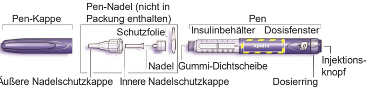
Schematische Zeichnung des Pens
