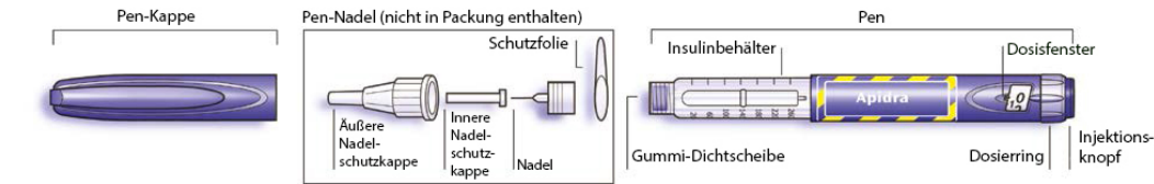
Schematische Zeichnung des Pens
