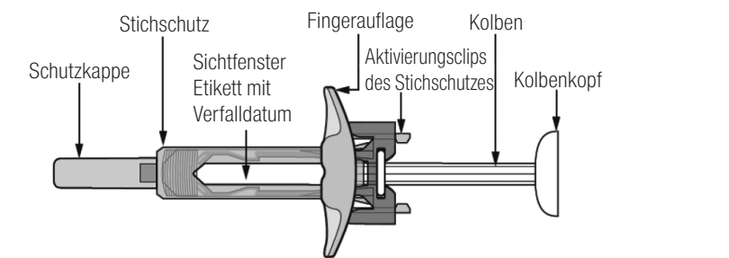
Abbildung A: Hyrimoz-Fertigspritze mit Stichschutz und Fingerauflage
