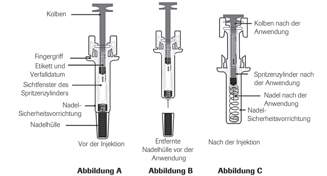
Abbildung A: Neue Spritze mit Nadelhülle Abbildung B: Neue Spritze ohne Nadelhülle Abbildung C: Spritze nach der Anwendung mit aktivierter Sicherheitsvorrichtung
