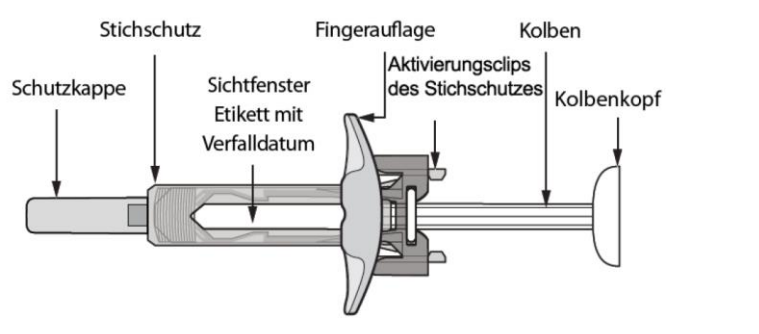
Abbildung A: Hyrimoz-Fertigspritze mit Stichschutz und Fingerauflage
